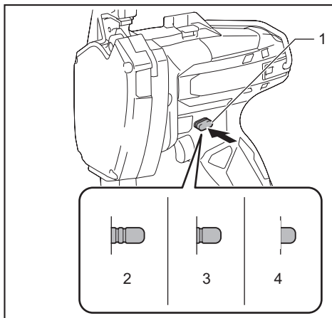
► 1. Levier inverseur 2. Position de découpe 3. Position verrouillée 4. Position d'inversion
