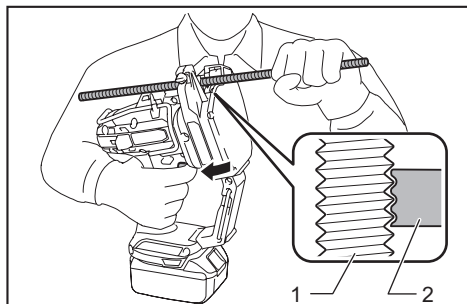
► 1. Tige filetée 2. Matrice de découpe sur la monture immobile
