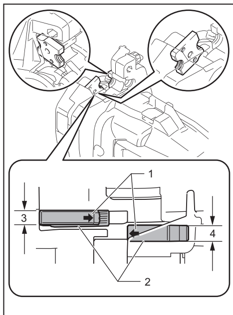
► 1. Flèche 2. Matrice de découpe 3. Côté mince 4. Côté épais
