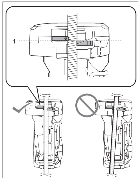
► 1. Ligne de coupe
