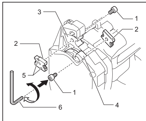
► 1. Boulon 2. Matrice de découpe 3. Monture immobile 4. Monture mobile 5. Marque colorée 6. Clé hexagonale
