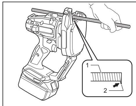
► 1. Tige filetée 2. Buvure
